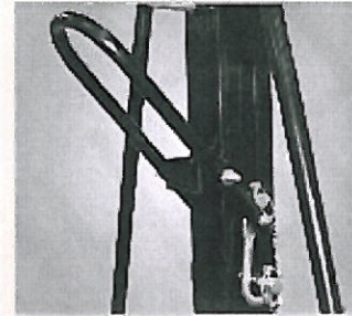
Einfache und sichere Höhenverstellung über Hebel und zwei Sicherungsbolzen
